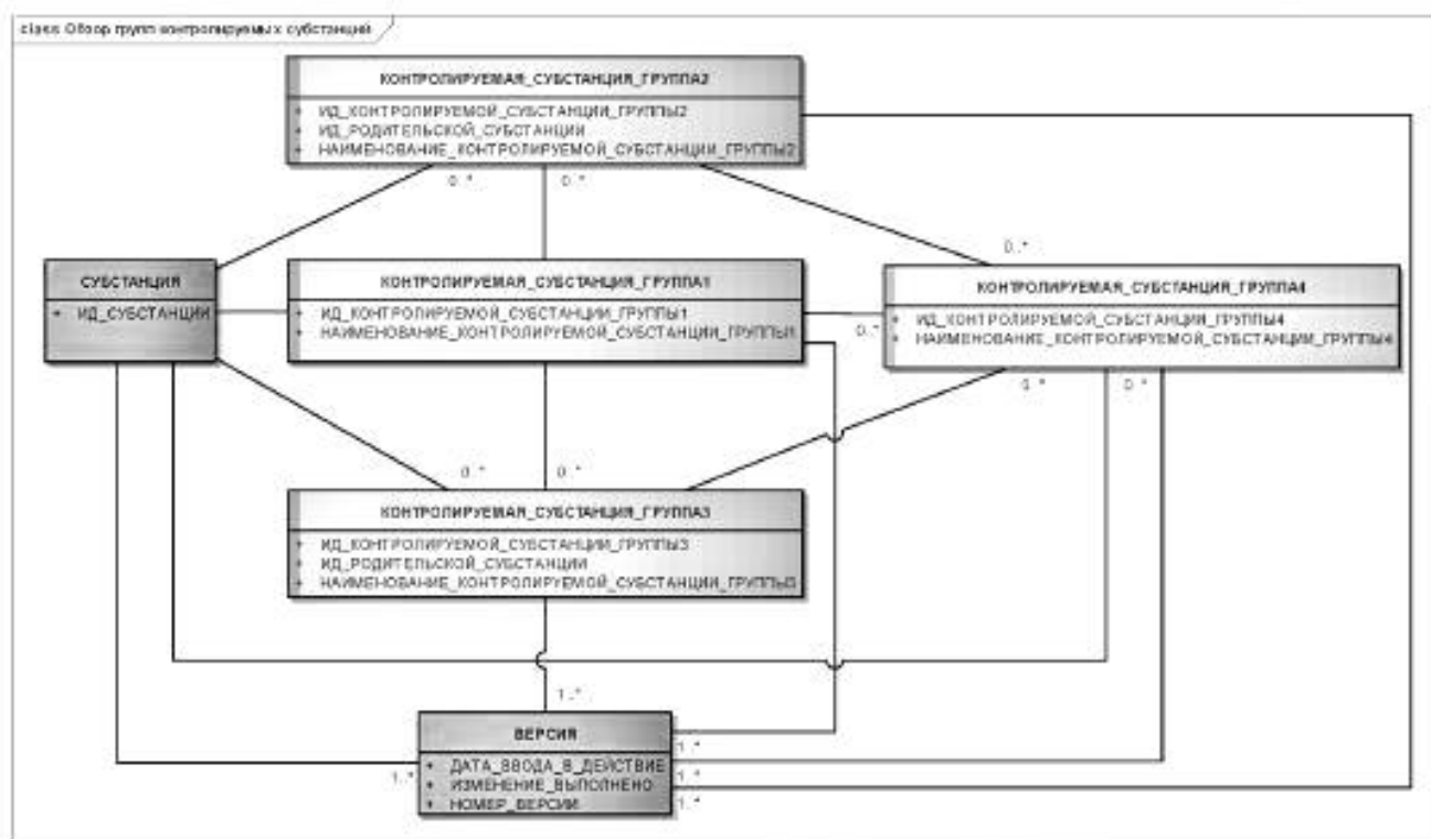
Рисунок 2 — Высокоуровневая информационная модель контролируемой субстанции
