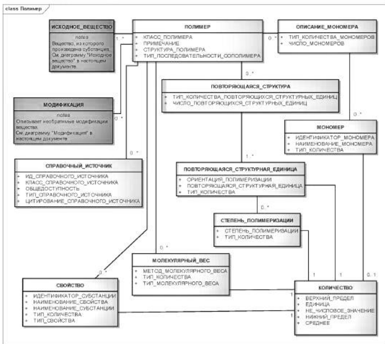
Рисунок 12 — Информационная модель описания полимера
