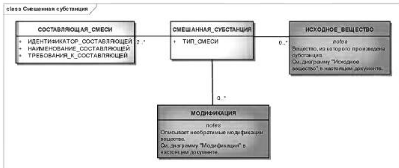
Рисунок 14 — Информационная модель описания смешанной субстанции
