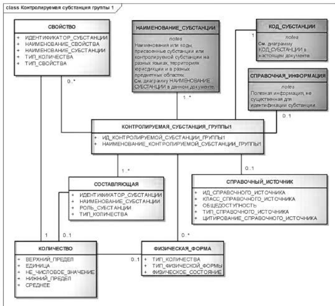
Рисунок 17 — Информационная модель описания контролируемой субстанции группы 1
