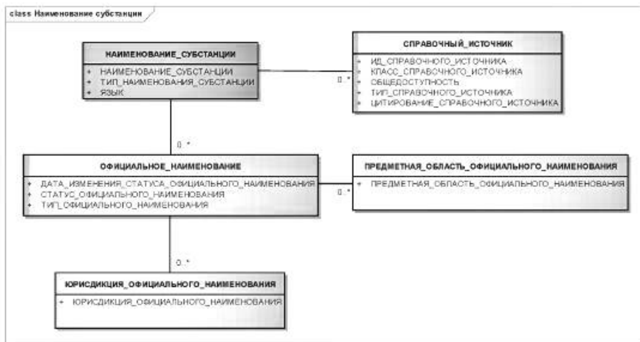
Рисунок 3 — Информационная модель наименований субстанции
