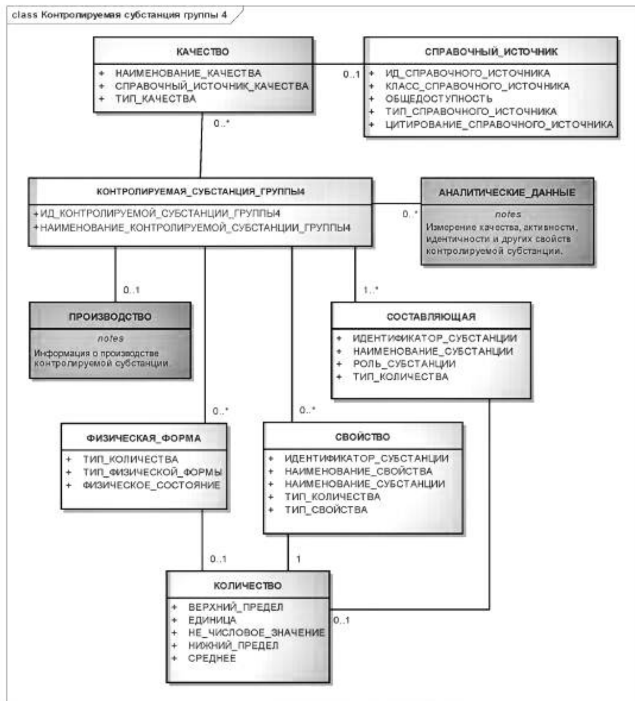
Рисунок 20 — Информационная модель описания контролируемой субстанции группы 4
