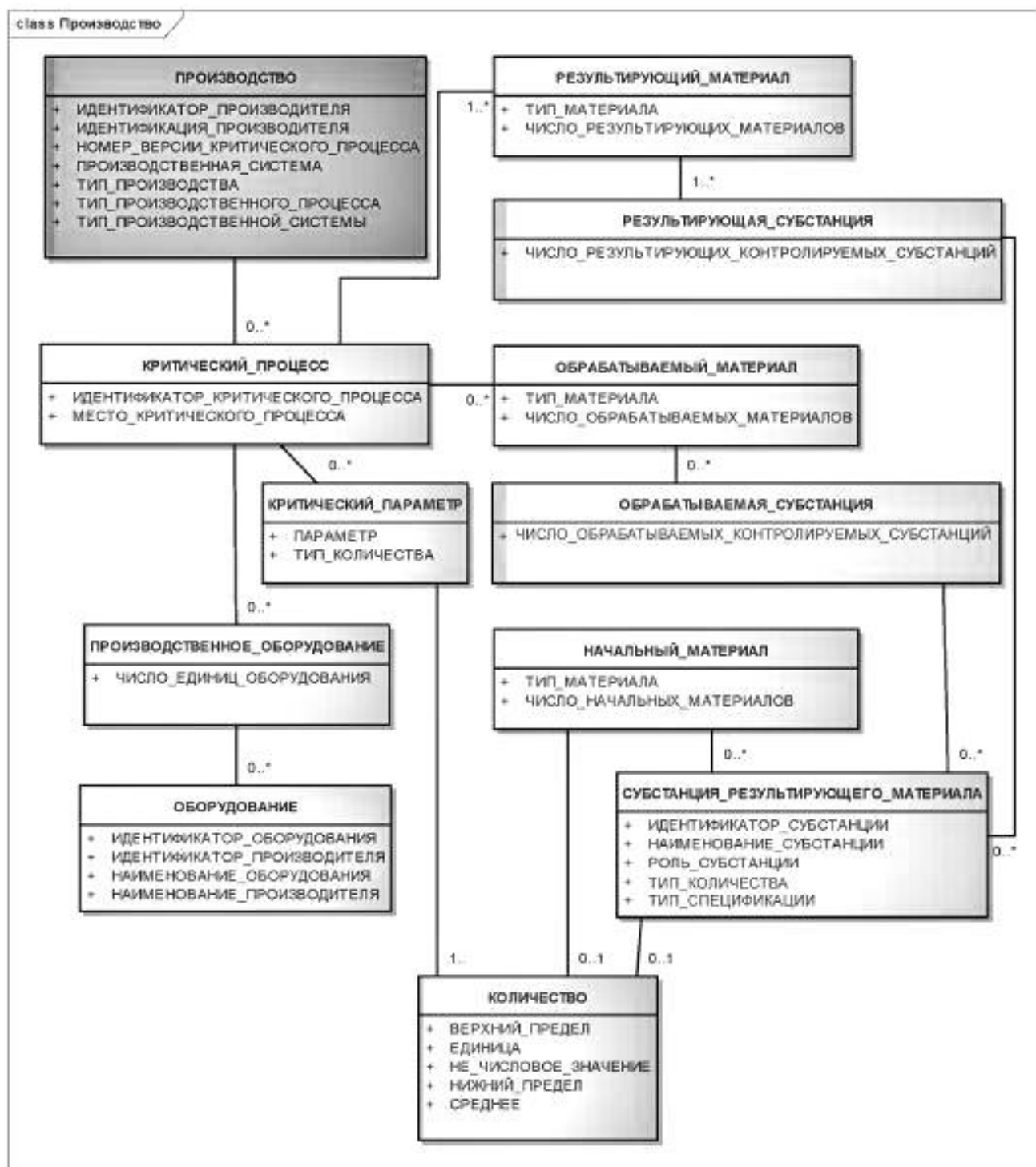
Рисунок 22 — Информационная модель описания производства
