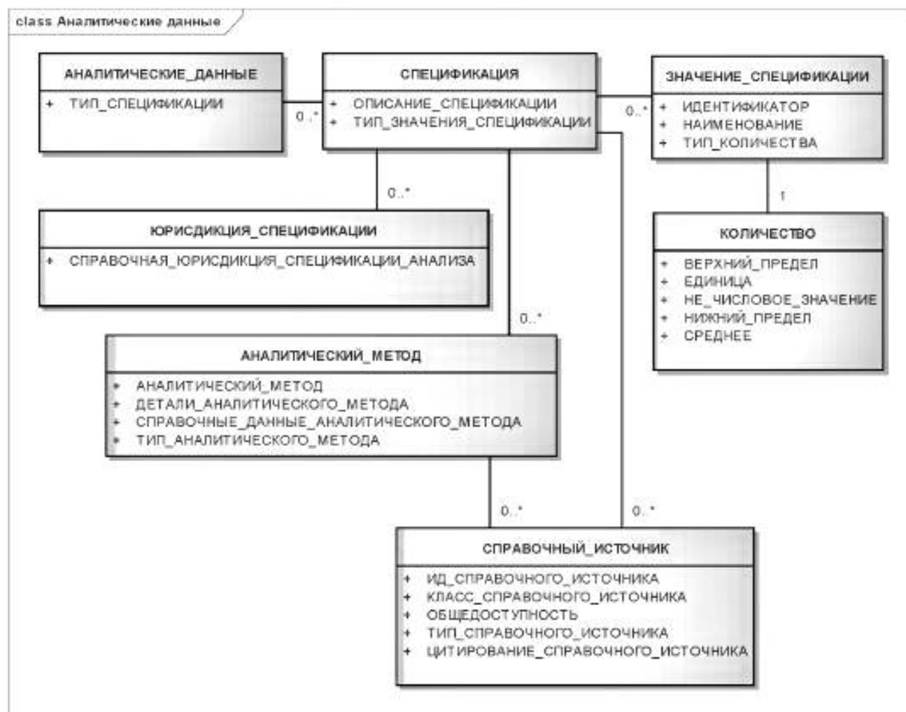
Рисунок 21 — Информационная модель описания аналитических данных
