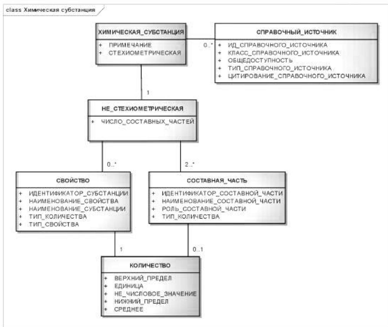
Рисунок 9 — Информационная модель описания химической субстанции
