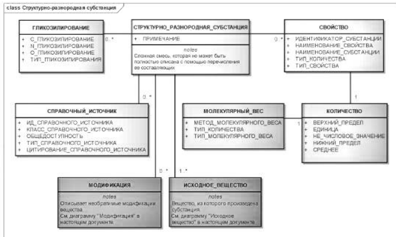
Рисунок 13 — Информационная модель описания структурно-разнородной субстанции
