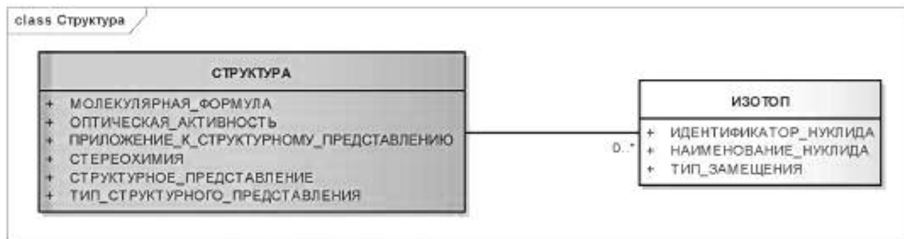
Рисунок 5 — Информационная модель описания структуры и изотопа
