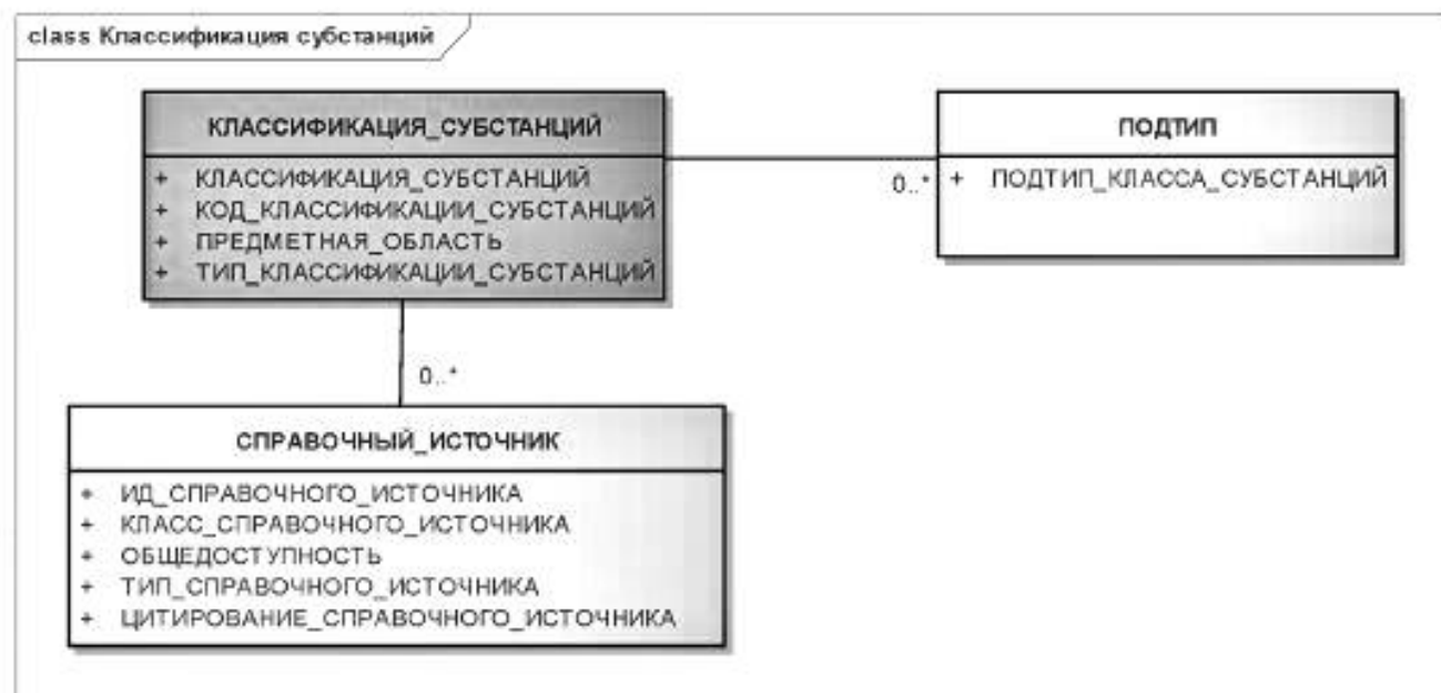
Рисунок 16 — Информационная модель классификации субстанций
