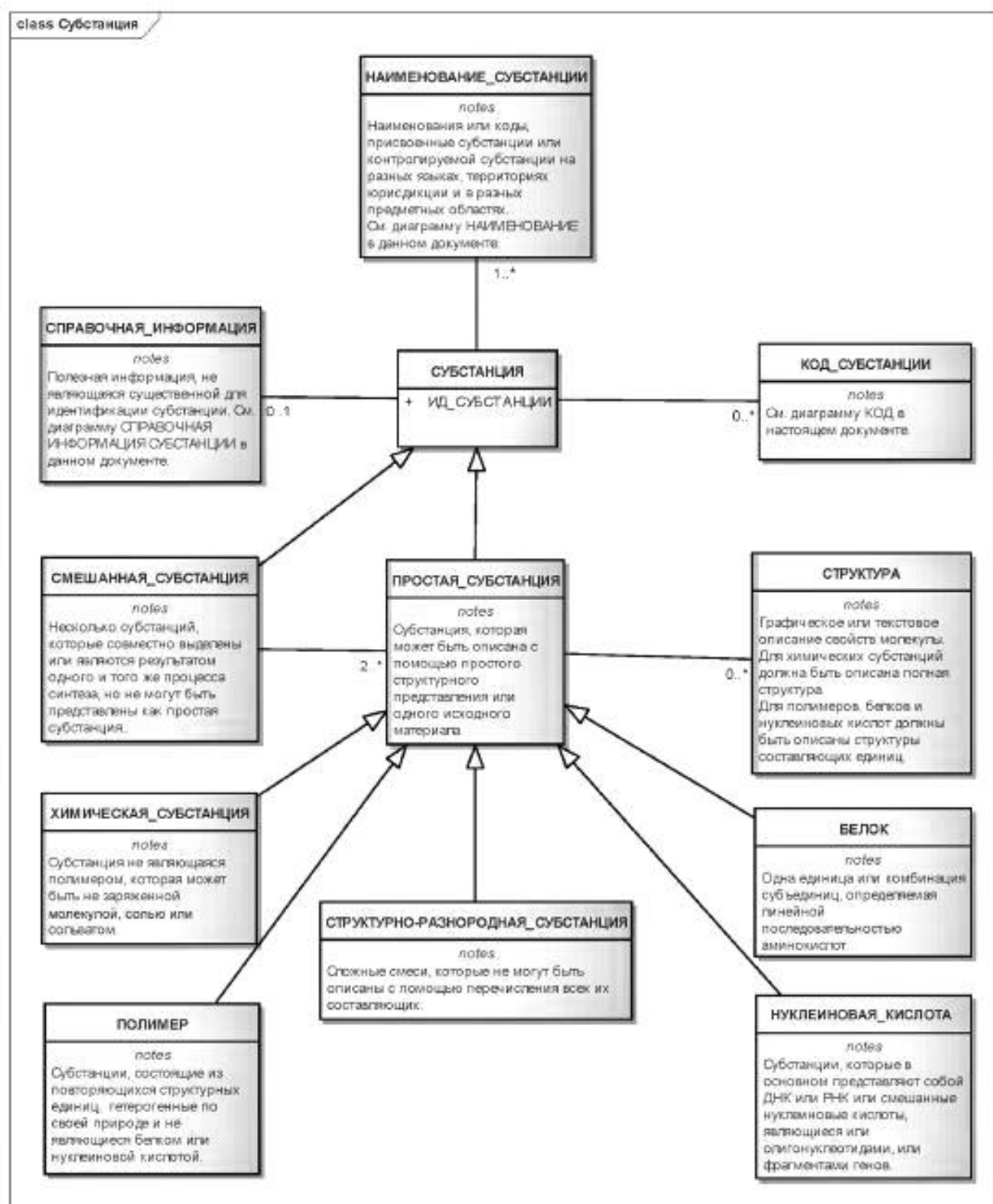
Рисунок 1 — Высокоуровневая информационная модель субстанции
