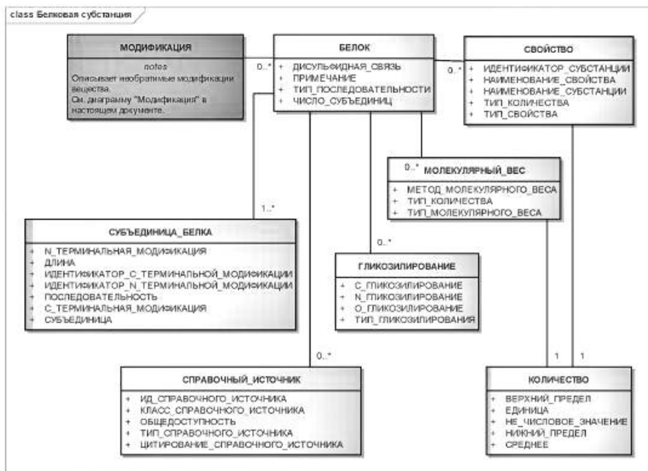
Рисунок 10 — Информационная модель описания белковой субстанции
