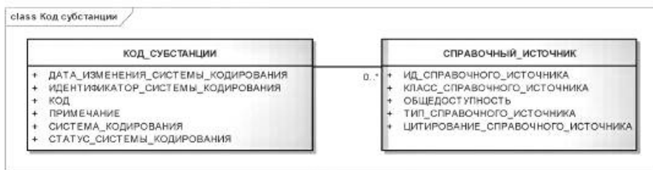
Рисунок 15 — Информационная модель кода субстанции
