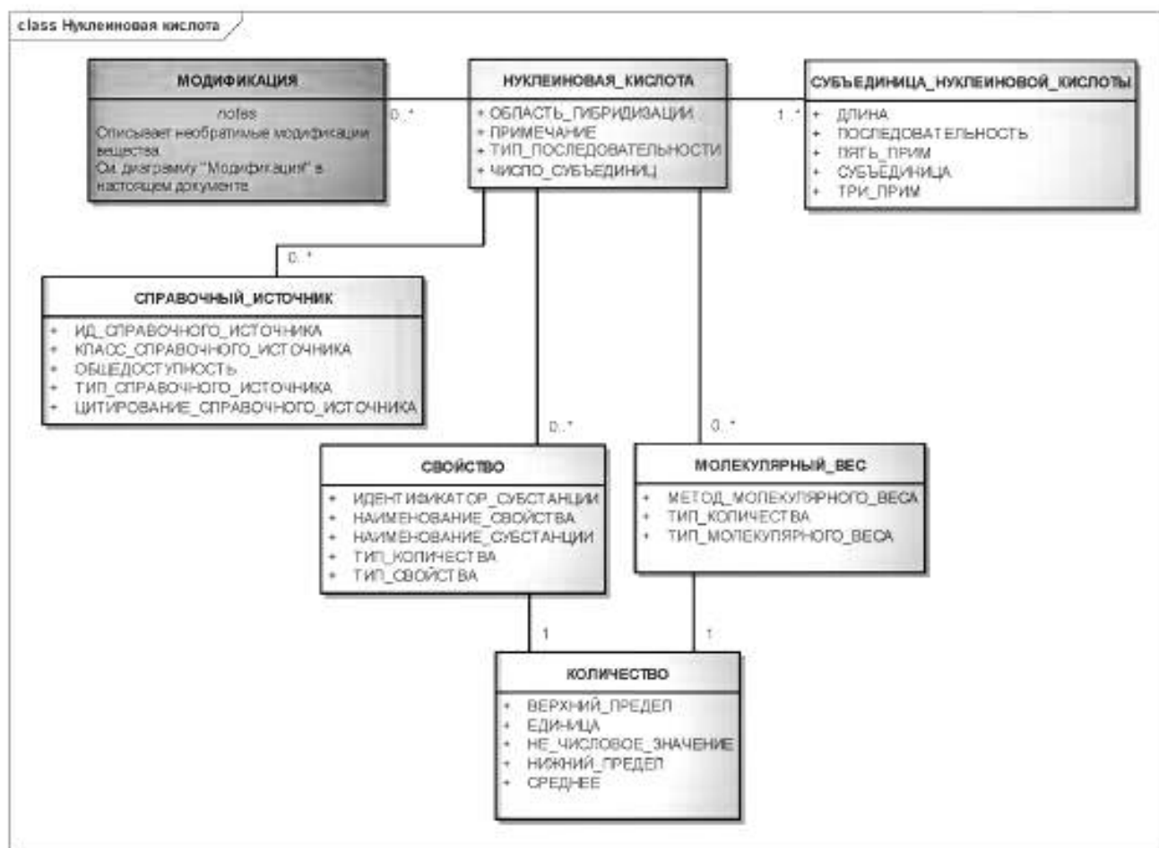
Рисунок 11 — Информационная модель описания нуклеиновой кислоты
