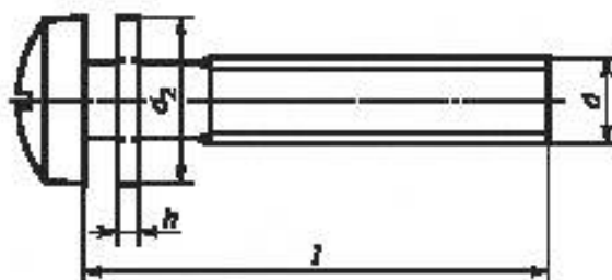
Рисунок 2 — Винт с уменьшенным стержнем
