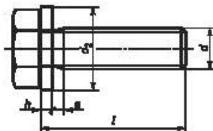
Рисунок 1 — Винт с резьбой, доходящей до шайбы
