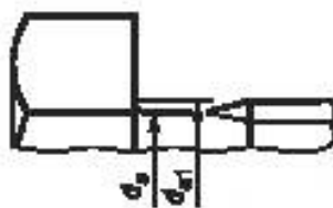
Рисунок 3 — Внутренний диаметр опорной поверхности d_{a1} и диаметр уменьшенного стержня d_s
