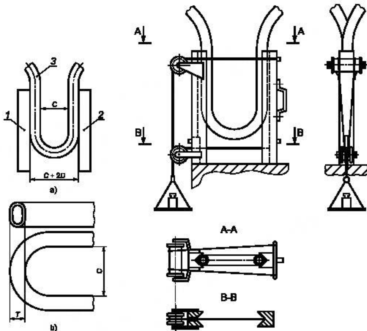
1 — направляющая А; 2 — направляющая В; 3 — испытуемый образец рукава
