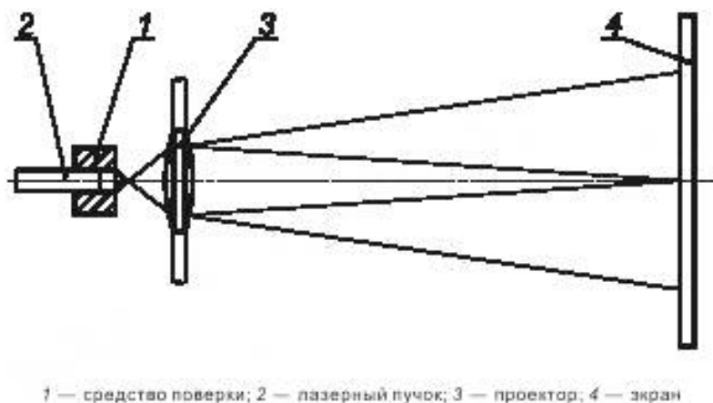
Рисунок А.2 — Схема проверки правильности установки эталонной линзы в восьмигранной оправе
