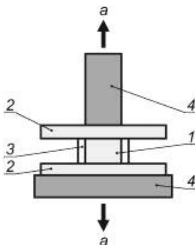
Рисунок 1 — Схема испытания на разрыв для измерения прочности соединения
